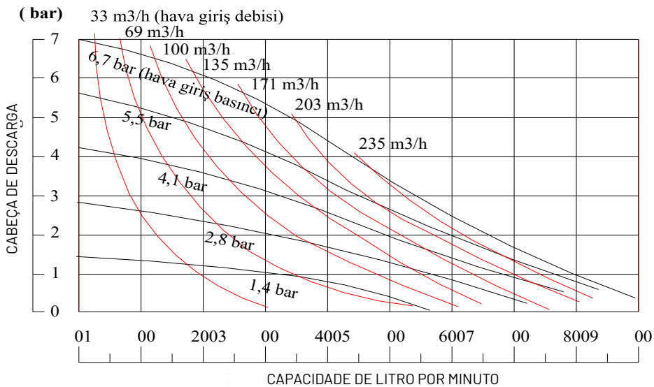
POLI FLOW - PX30 - CURVA DE DESEMPENHO
