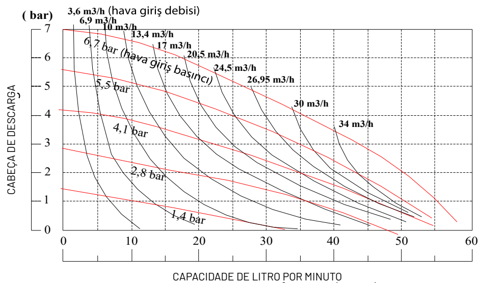
METALICFLOW - PX05 - CURVA DE DESEMPENHO
